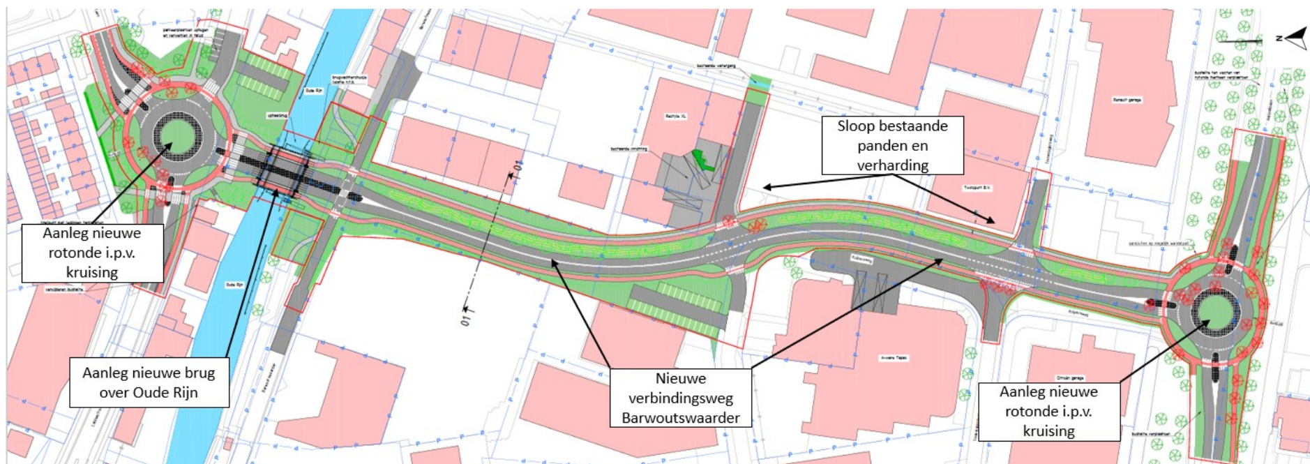
Afbeelding 4.2 Geplande inrichting van de te realiseren verbindingsweg
