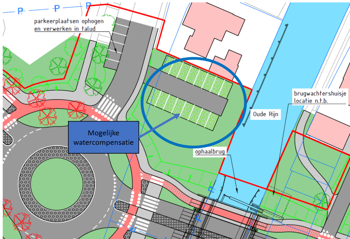
Afbeelding 4.5 Mogelijkheid voor inpassing van watercompensatie binnen het plangebied: ter plaatse van geplande parkeervoorzieningen
