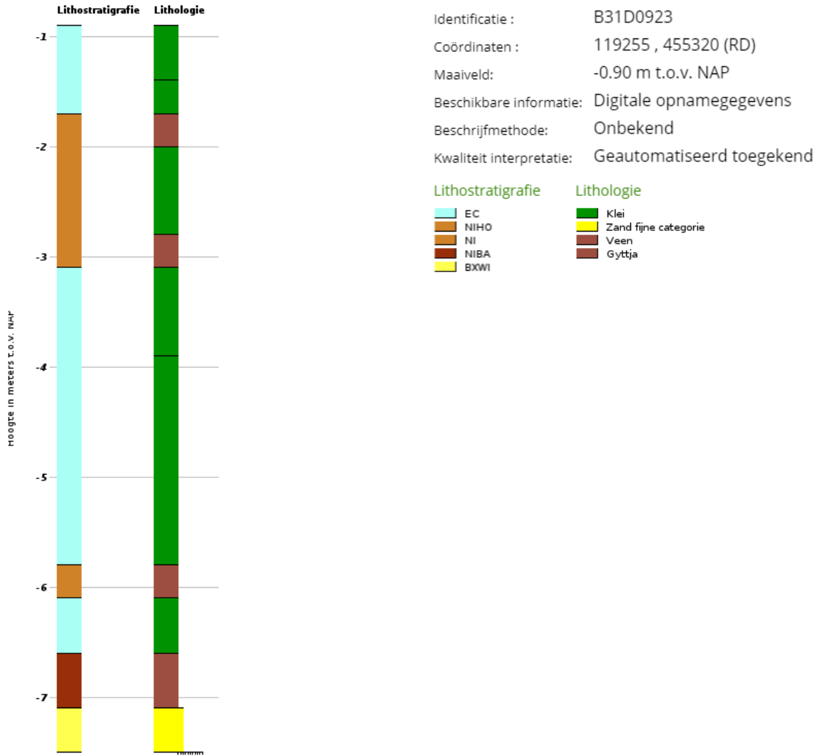
Afbeelding II.2 Boormonsterprofiel B31D0923 genomen aan de Barwoutswaarder/Hoge Rijndijk
