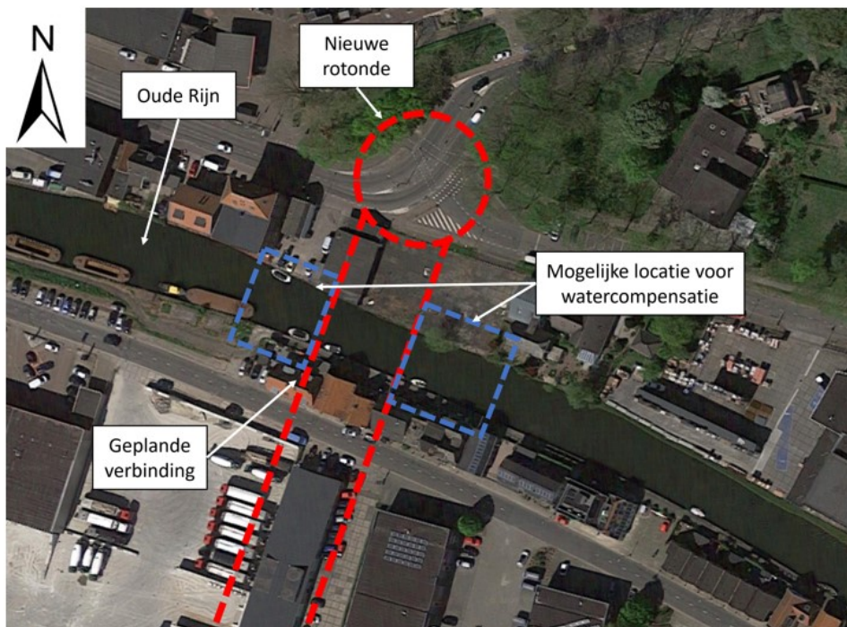
Afbeelding 4.4 Mogelijkheid voor inpassing van watercompensatie binnen het plangebied: profiel van de Oude Rijn verbreden
