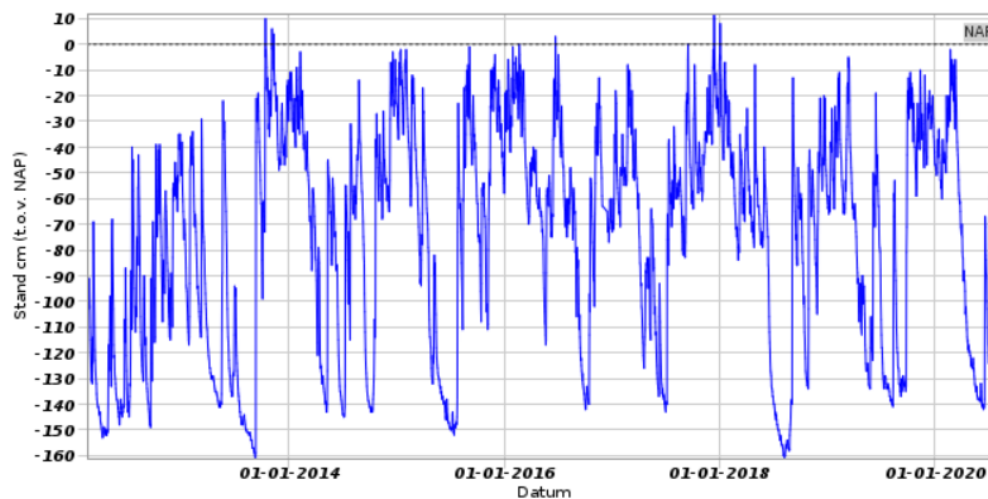
Afbeelding 3.5 Freatische grondwaterstand gemeten door peilbuis B31D1525 (Locatie 2) gemeten als functie van de tijd. Het maaiveld ligt op NAP +0,43 m
