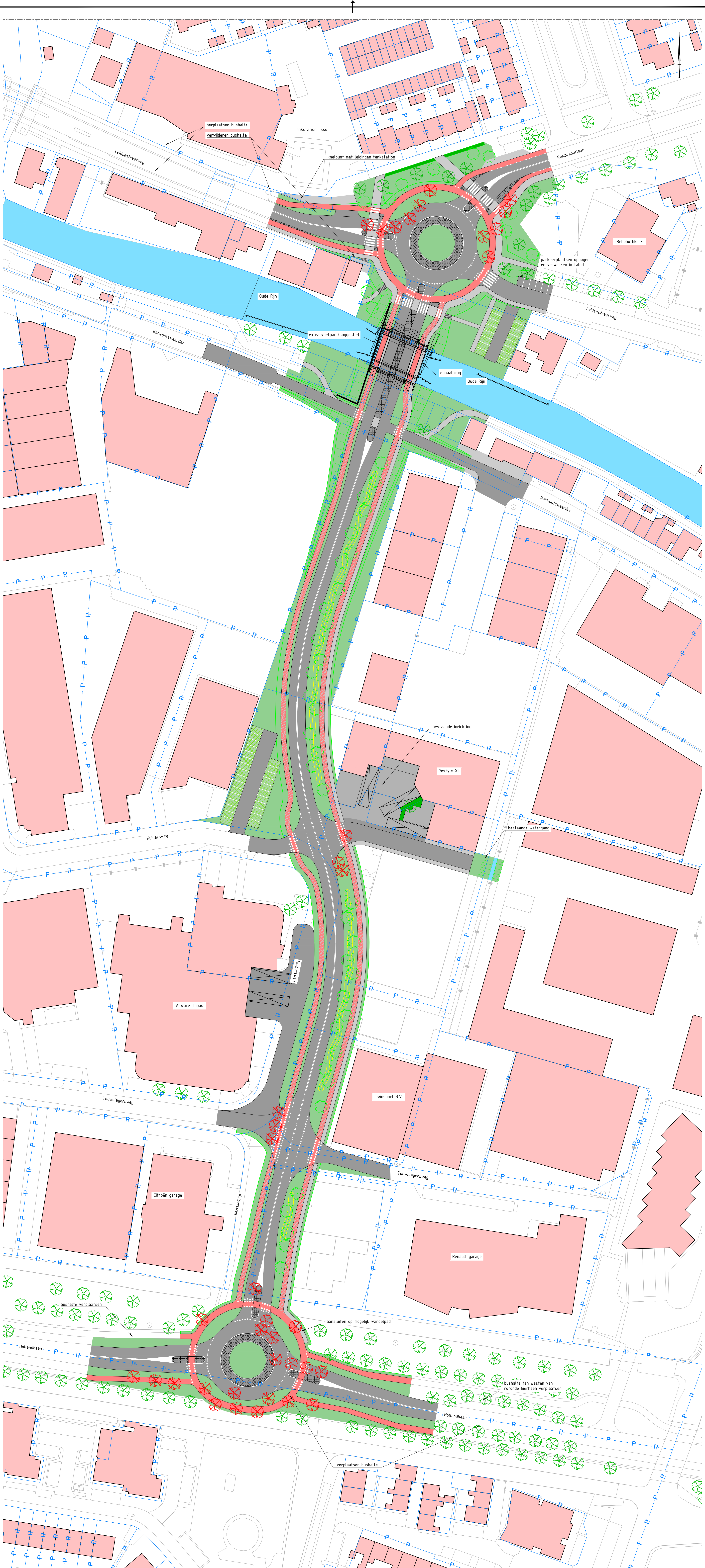
SITUATIETEKENING SCHAAL 1: 500
