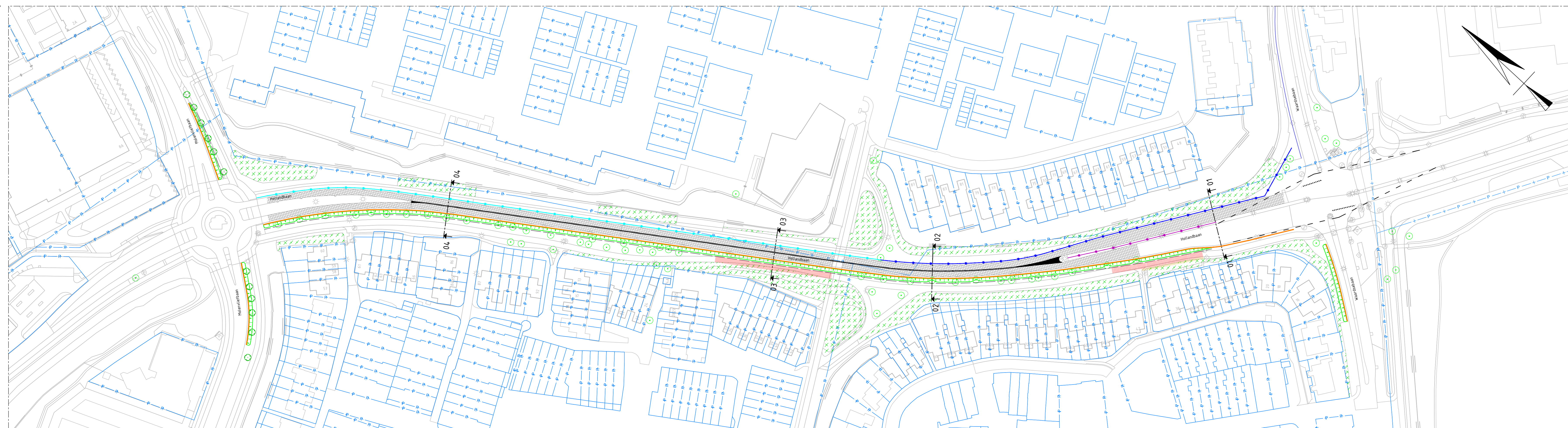
SITUATIETEKENING VARIANT 2 (SCHANSKORF MET GROEN AANZICHT DMV GRONDWAL) SCHAAAL 1:1000
