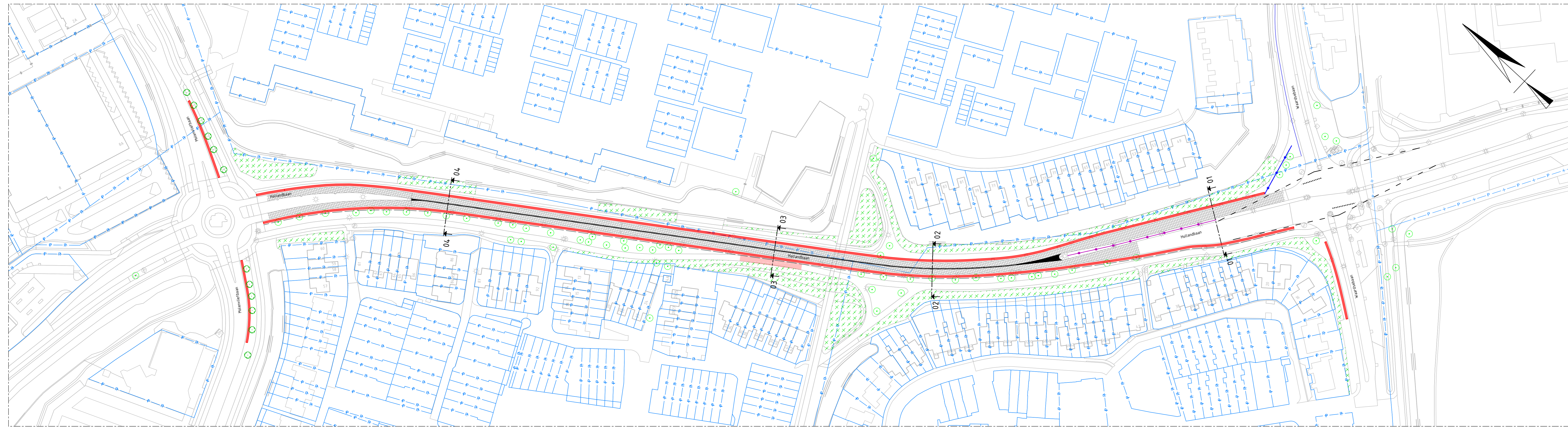
SITUATIETEKENING VARIANT 1 (WHISWALL) SCHAAAL 1:1000
