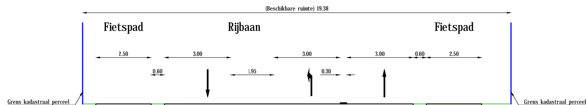
Principe dwarsprofiel A-A VRI kruispunt Schaal 1:100
